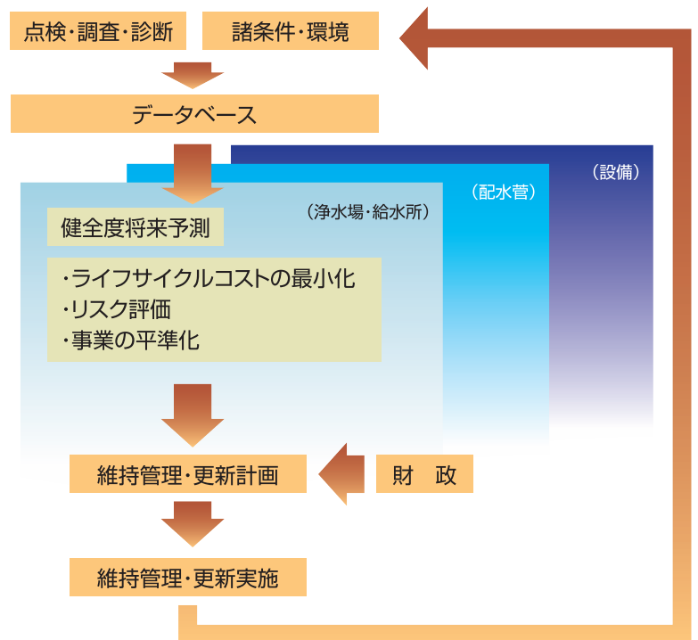
水道施設のアセットマネジメントフロ (イメージ図)
